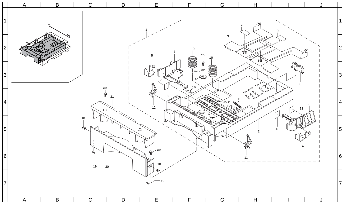
FIG. 2 CASSETTE
